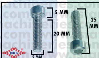
A11/B15 BAUT VORING M5X20 CS5200/5800
