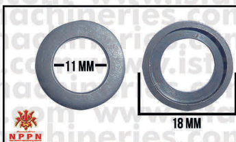
A38 WASHER CS5200/5800
