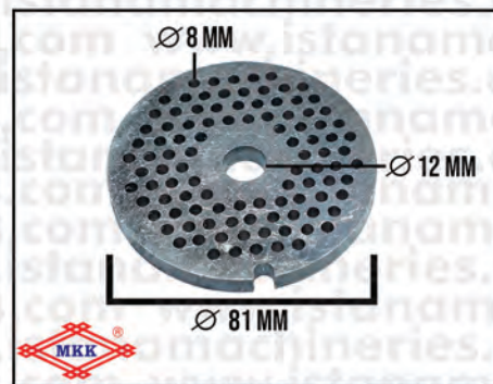
SARANGAN/PISAU GILINGAN DAGING 22 INCH 8MM
