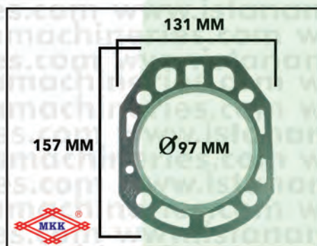
GASKET HEAD 2MM D185
