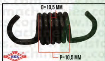
CLUTCH SPRING 3WZ4/TU26
