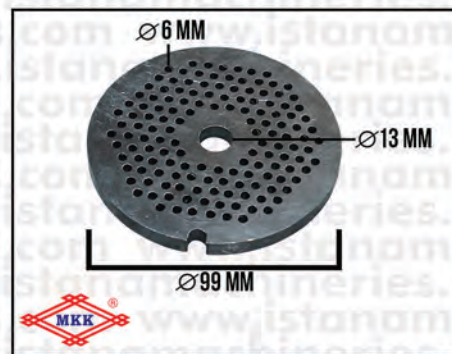
SARANGAN/PISAU GILANGAN DAGING 32 INCH 6 MM
