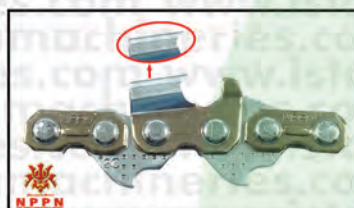
RANTAI 3/8 0.058 38MT (BULAT)
