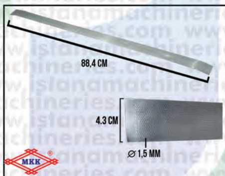
SARANGAN FFC23 1,5 MM
