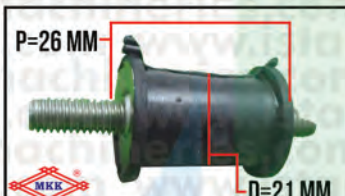
KAKI MESIN "PANJANG" 3WZ4/TU26
