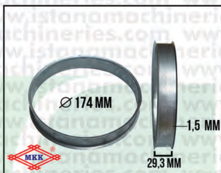
SARANGAN 1,5 MM FFC15
