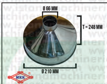
CORONG GILINGAN KEDELAI 8"
