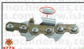
RANTAI 3/8 0.058 34MT (BULAT)
