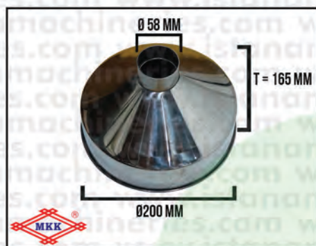
CORONG GILINGAN KEDELAI 6"
