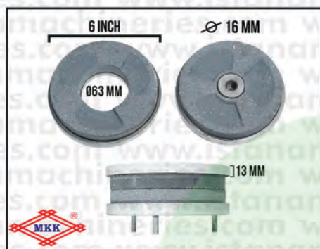
BATU ASSY GILINGAN CABAI 6" PMJA
