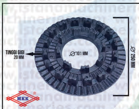
GIGI PINTU/TOOTH DISC FFC23
