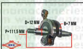
CRANKSHAFT 33 3WZ4/TU26
