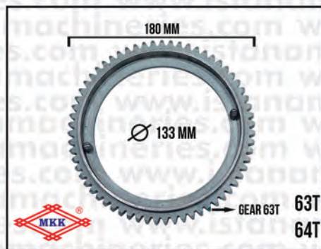
BIG GEAR N50
