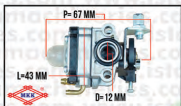
CARBURATORR "MODEL MEMBRANE" 867/869
