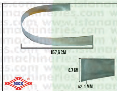
SARANGAN FFC45 1 MM
