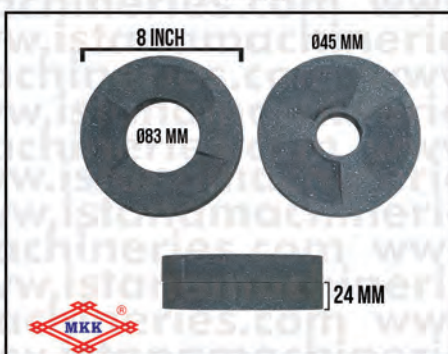
BATU ONLY GILINGAN CABAI 8" PMJA
