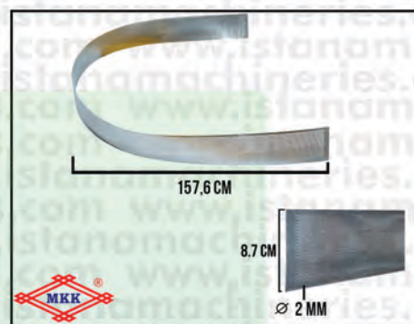
SARANGAN FFC45 2 MM
