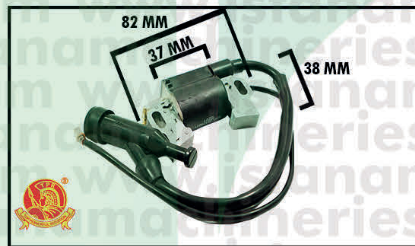
C.D.I W/COP BUSI GX270>420/ET8000ES
