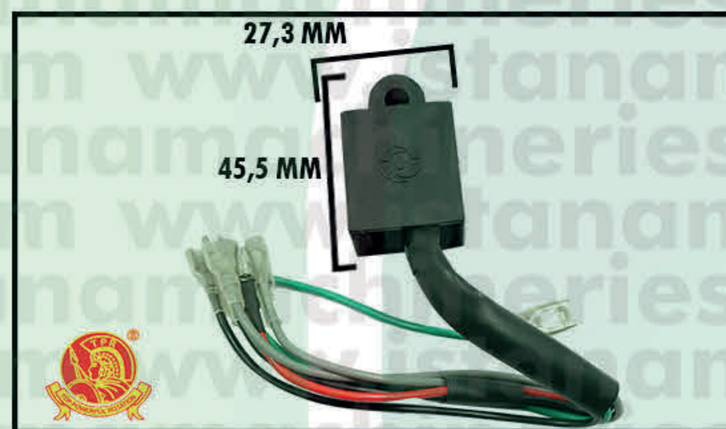
C.D.I ET950
