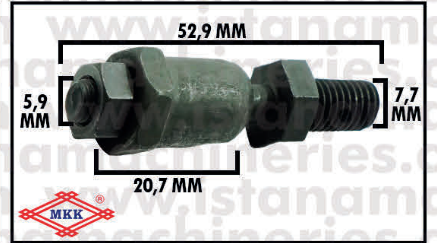
BOLT+PIVOT+NUT GX110 > 200
