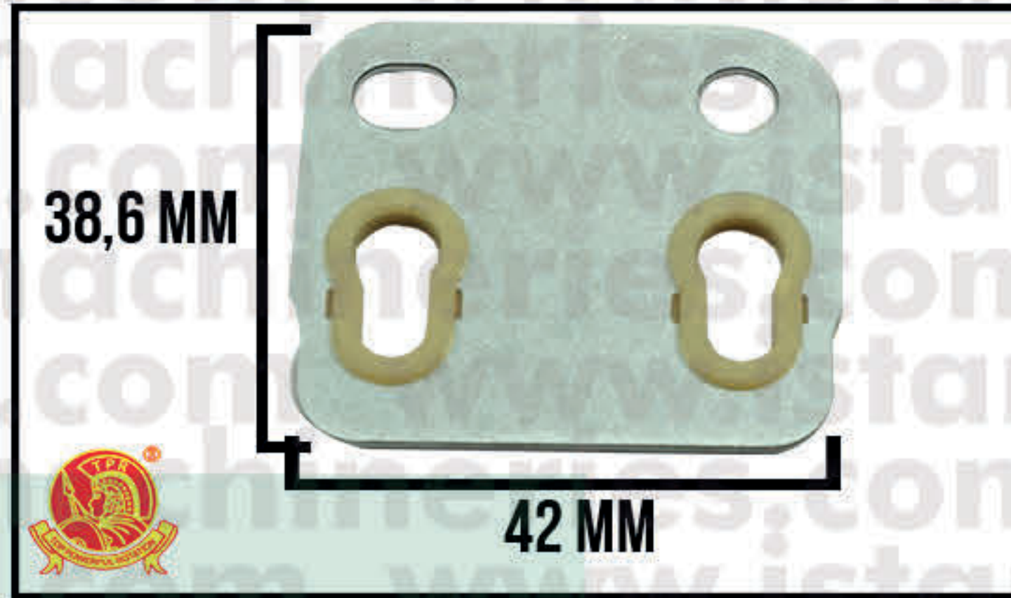
PLAT PUSH ROD ET1500
