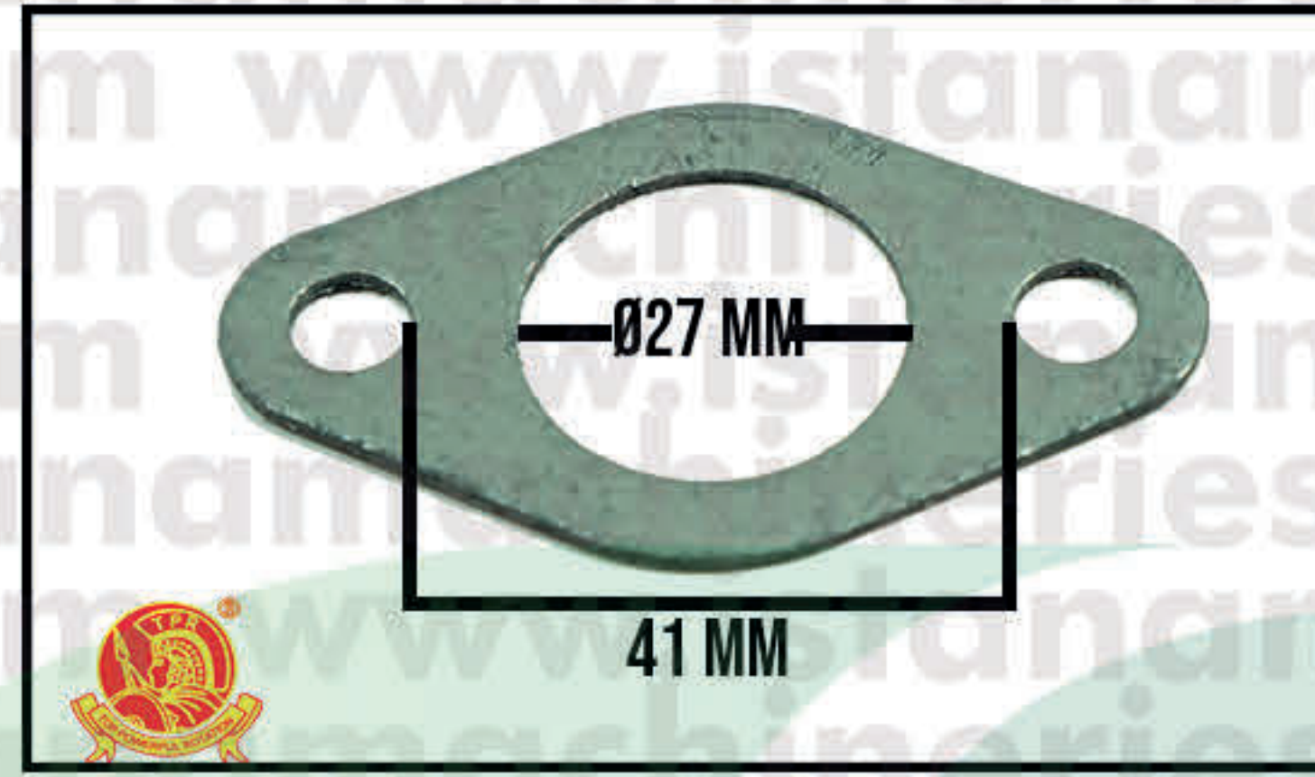
PACKING KNALPOT GX270
