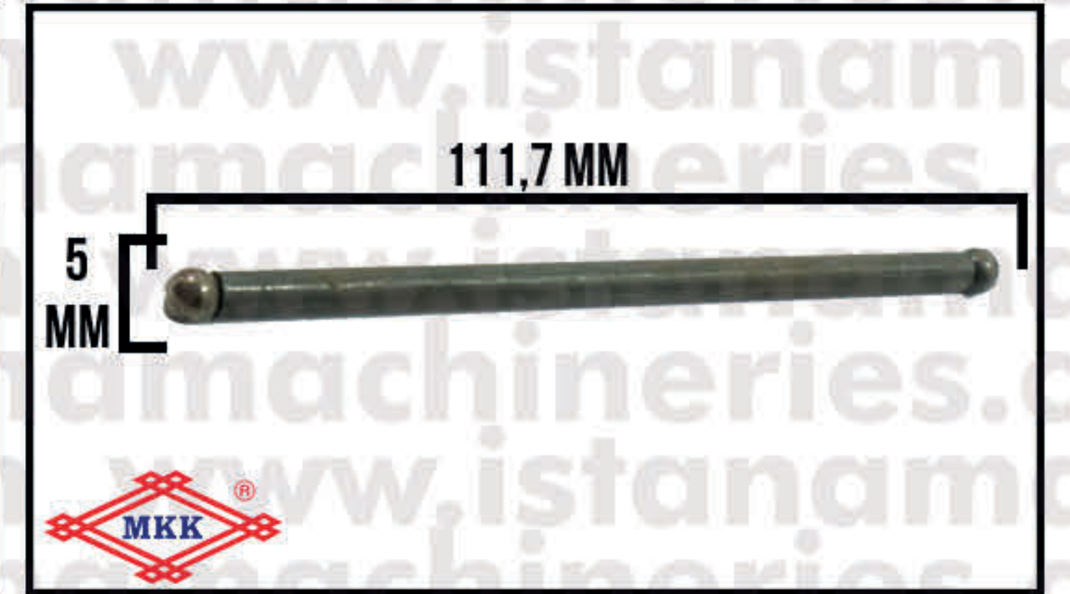
PUSH ROD ET-1500
