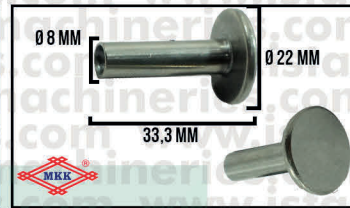
TAPPET ET-1500
