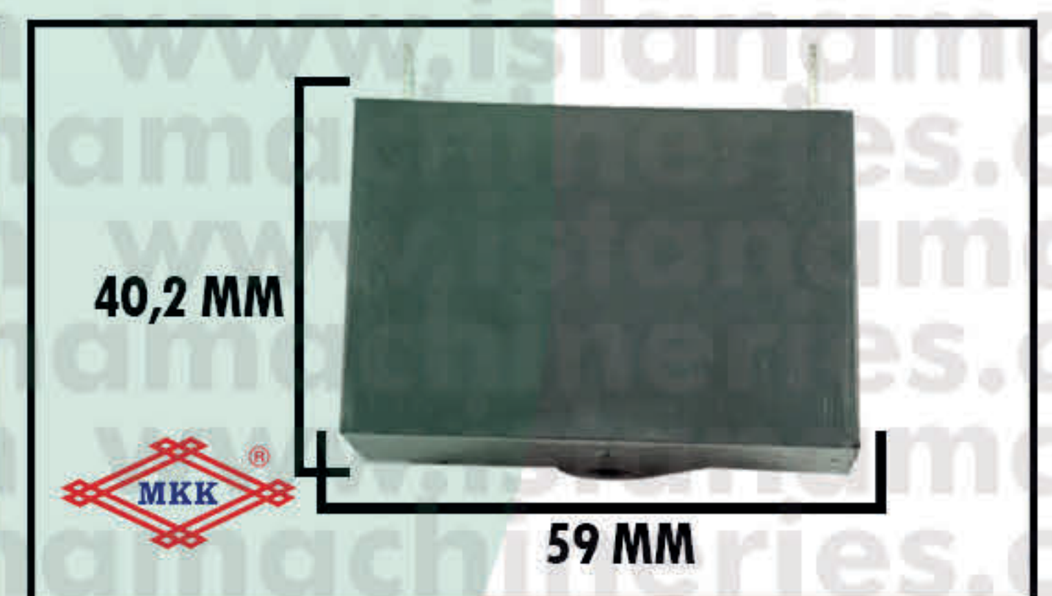
CAPACITOR SEGI 24 UF 350VA ET950
