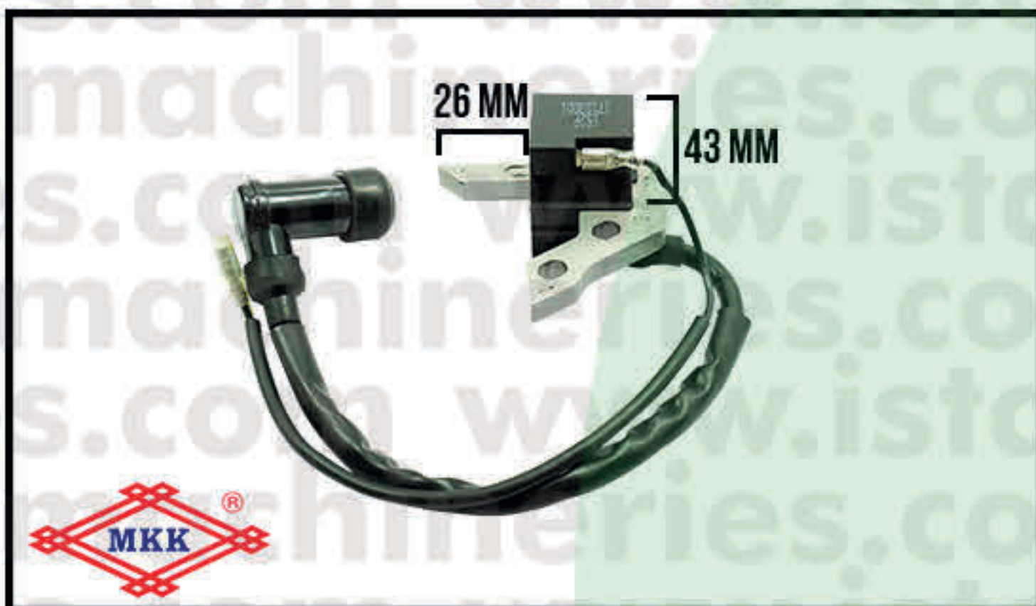
C.D.I "BODY KECIL" ET1500
