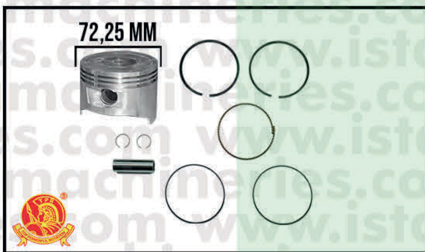
PISTON ASSY 0,25 GX270
