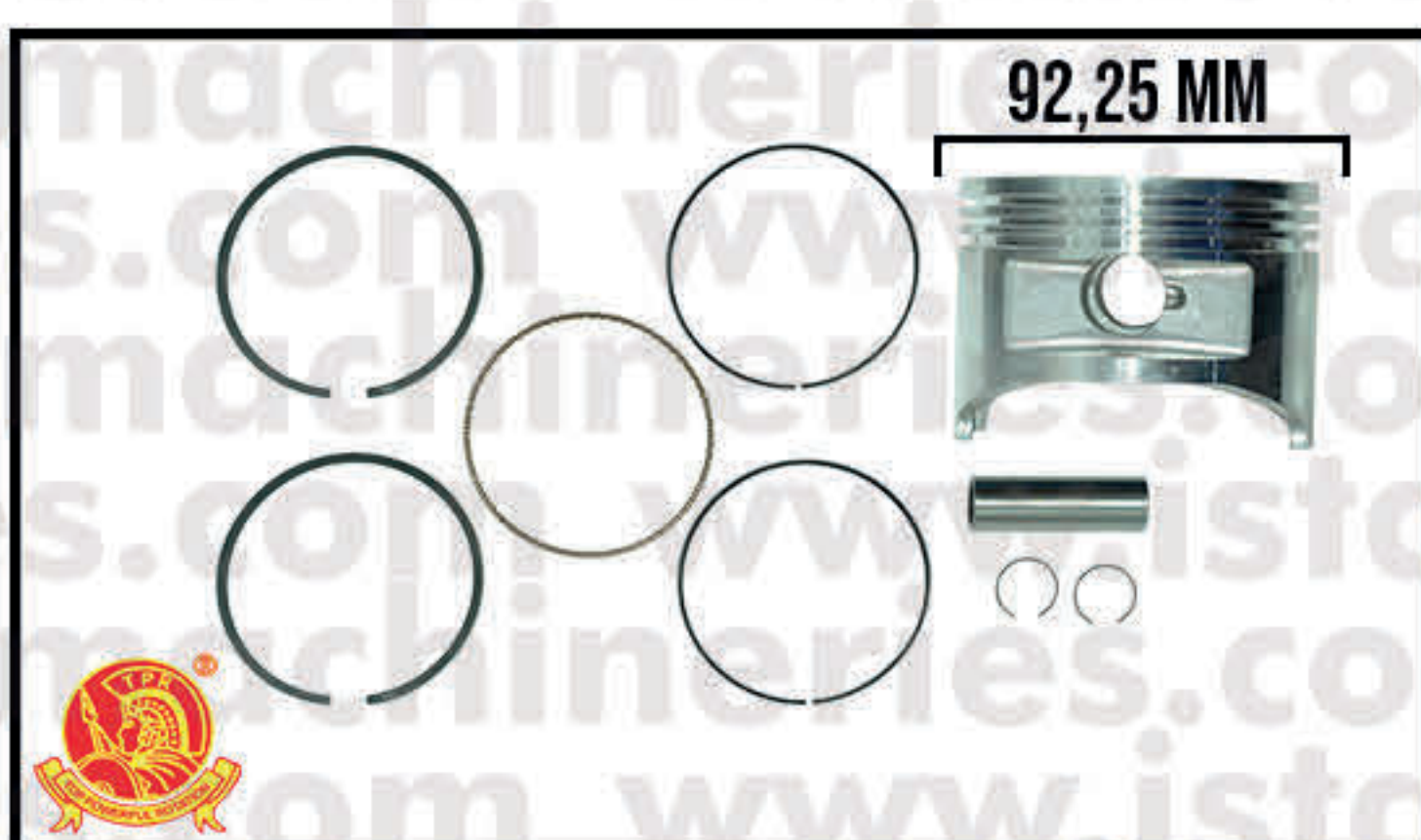
PISTON ASSY 0,25 GX460
