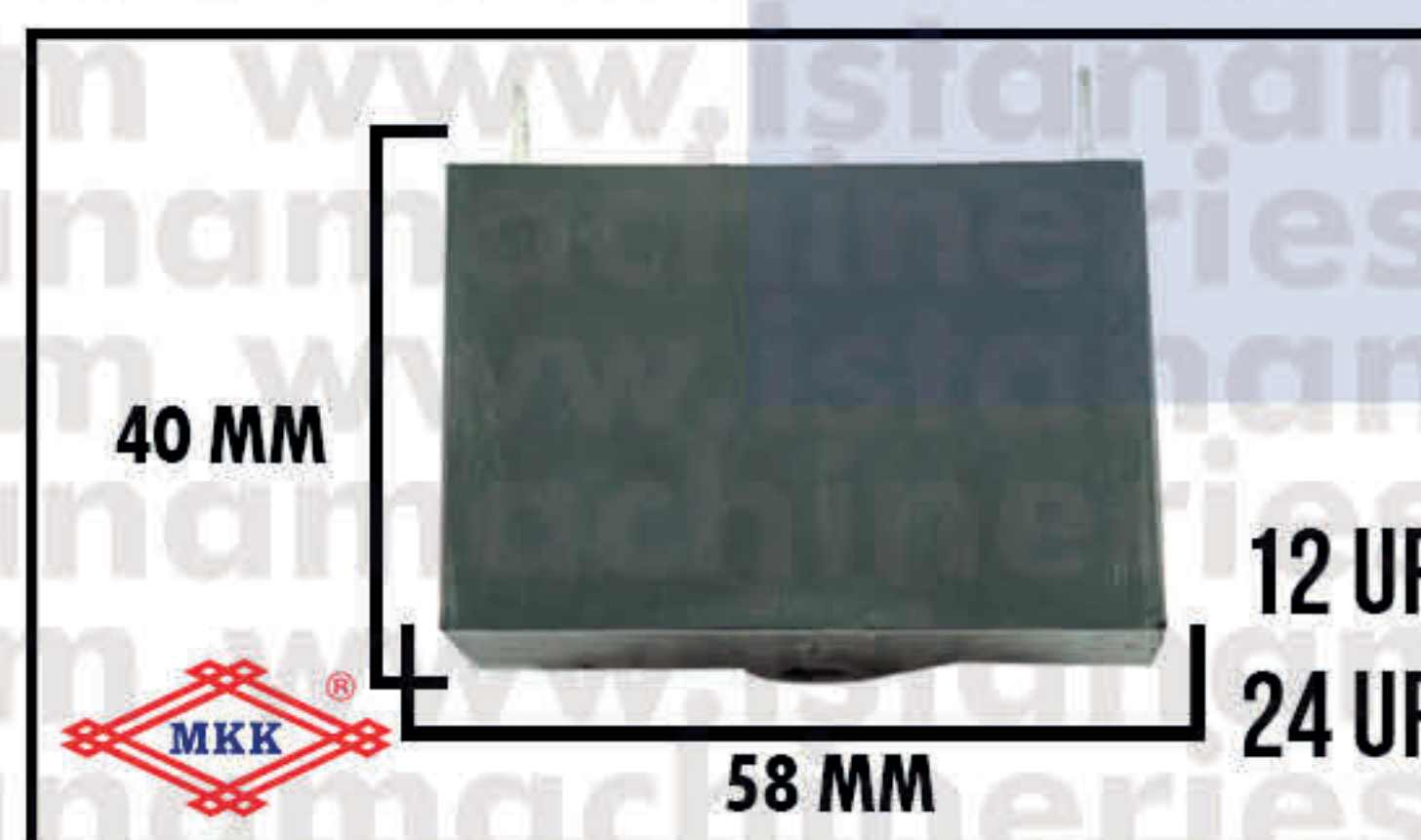
CAPACITOR SEGI 24 UF 450VA ET950
