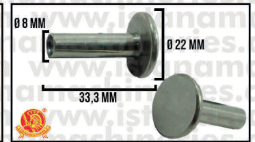
TAPPET ET 1500
