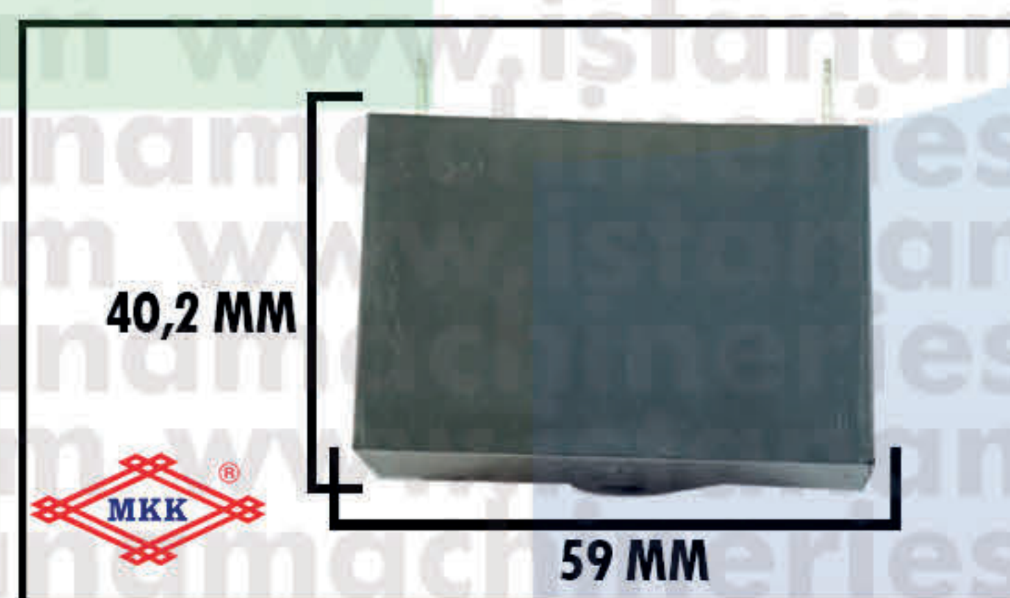
CAPACITOR SEGI 15 UF 350VA ET950
