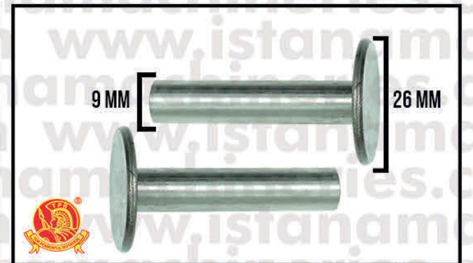
TAPPET GX390>460
