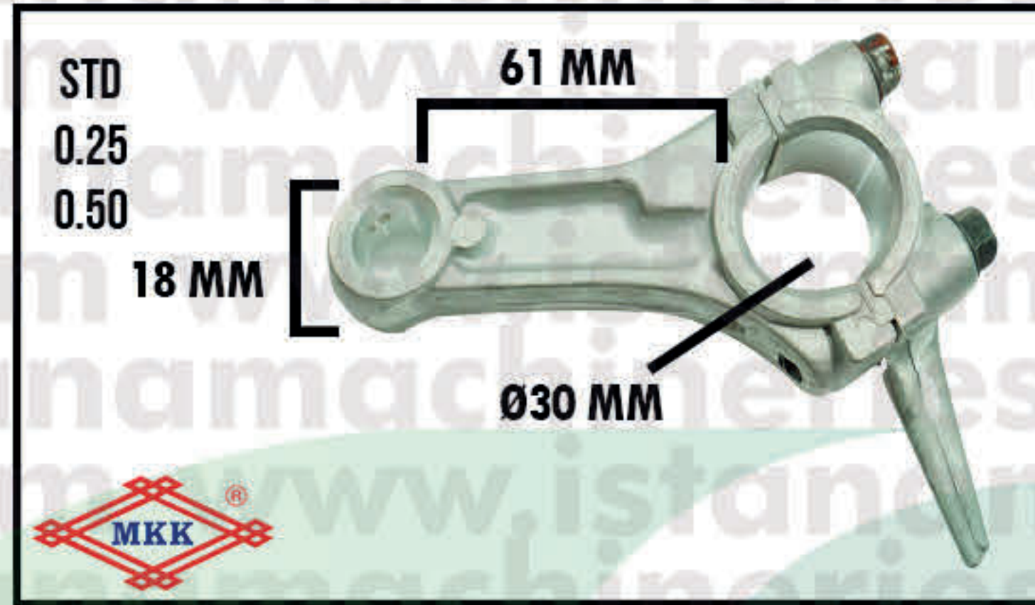
CONROD GX140 > 200
