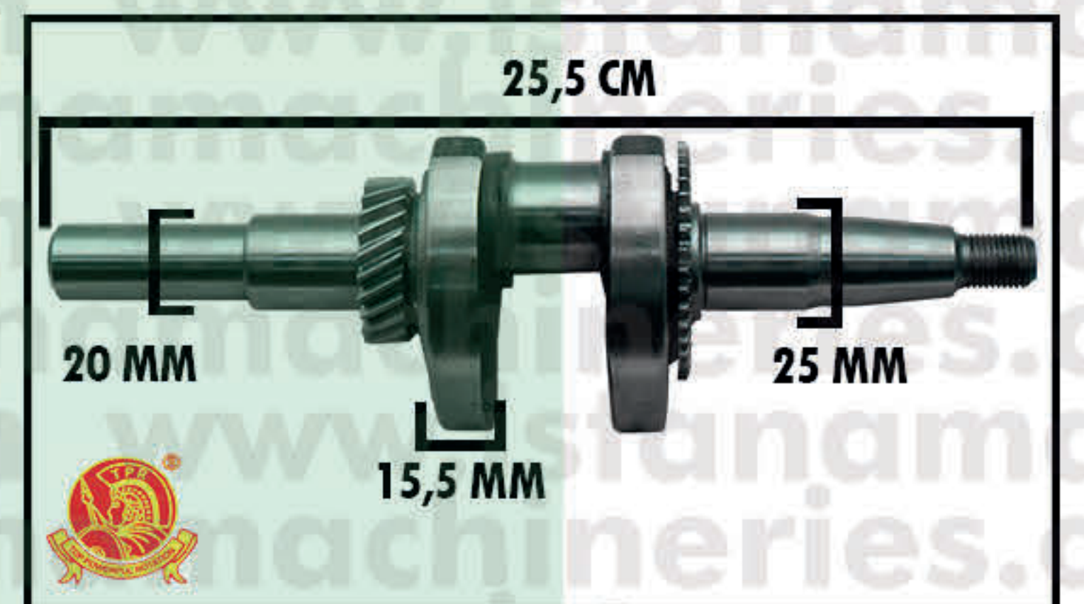
CRANKSHAFT "DRAT-SPIE" GX140/160
