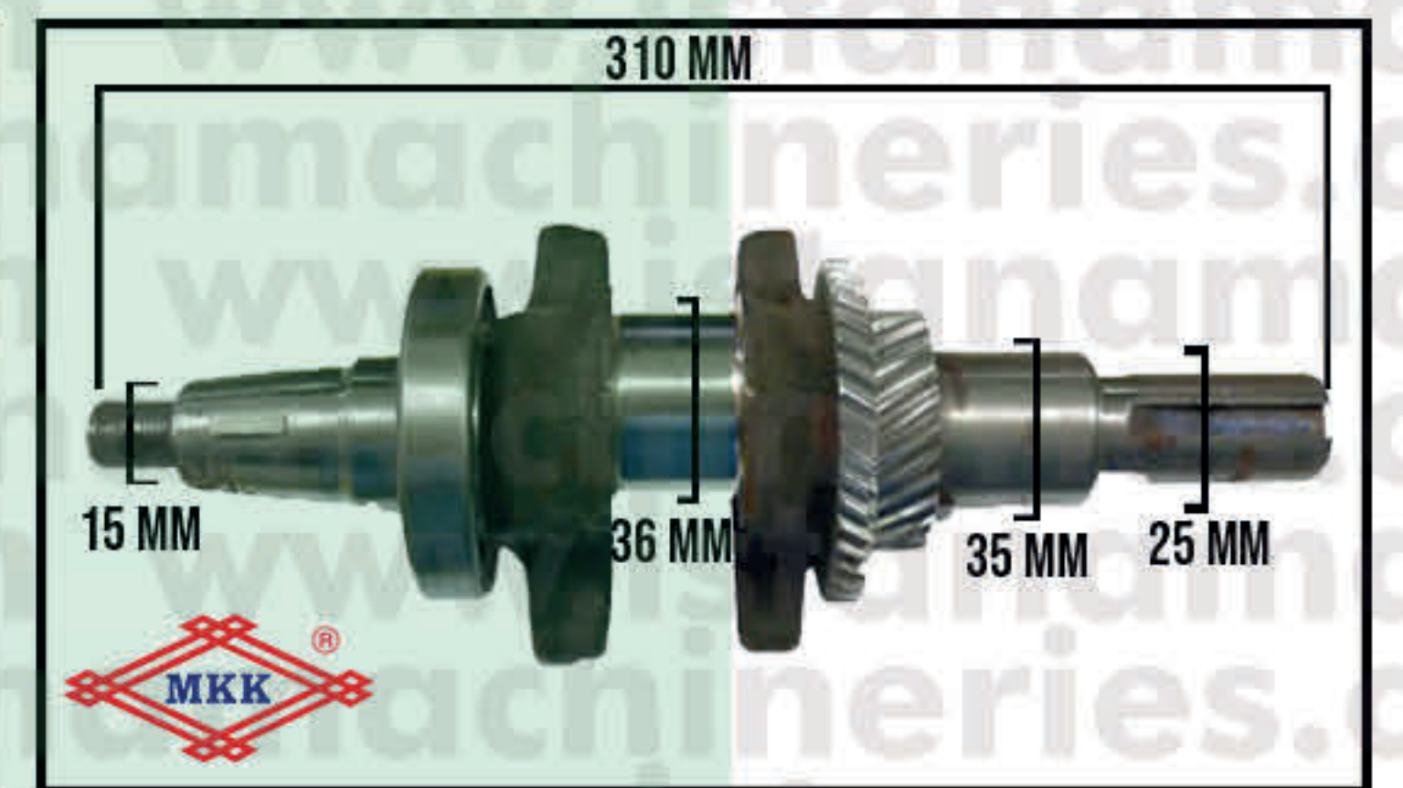
CRANKSHAFT SPIE GX390>420
